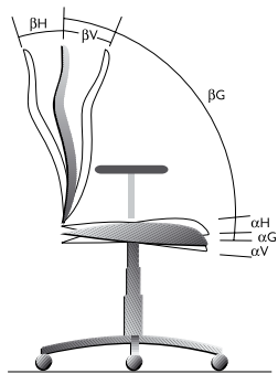
Ergonomisch relevante Sitzmaße und -winkel
