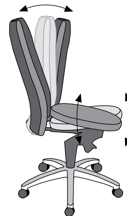
Stuhl mit Synchronablauf von Sitz- und Lehnenfläche sowie mit Bewegungsmöglichkeiten der Sitzfläche am Beispiel ERGO TOP
